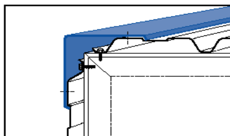
VONKAJŠÍ ROHOVÝ SPOJ
