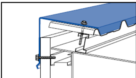
HREBENÁČ PULTOVEJ STRECHY
