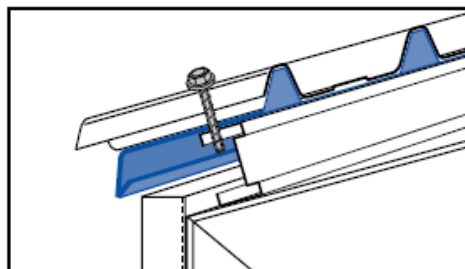
PROFILOVANÝ UZATVÁRACÍ PLECH
