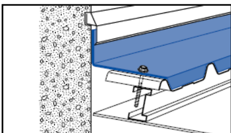
PRIEČNA LEMOVKA NA FASÁDU
