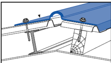
POLOVIČNÝ HREBENÁČ S FALCOM
