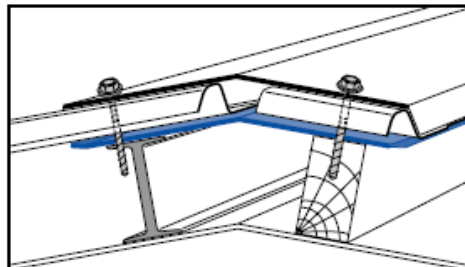
HREBENÁČ POD PLECHOM
